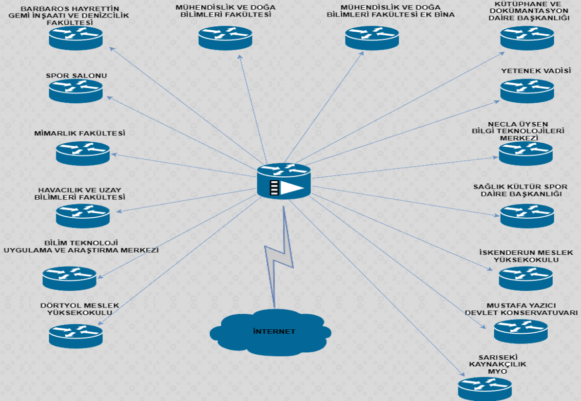
Şekil 1. İskenderun Teknik Üniversitesi Ağ Topolojisi
